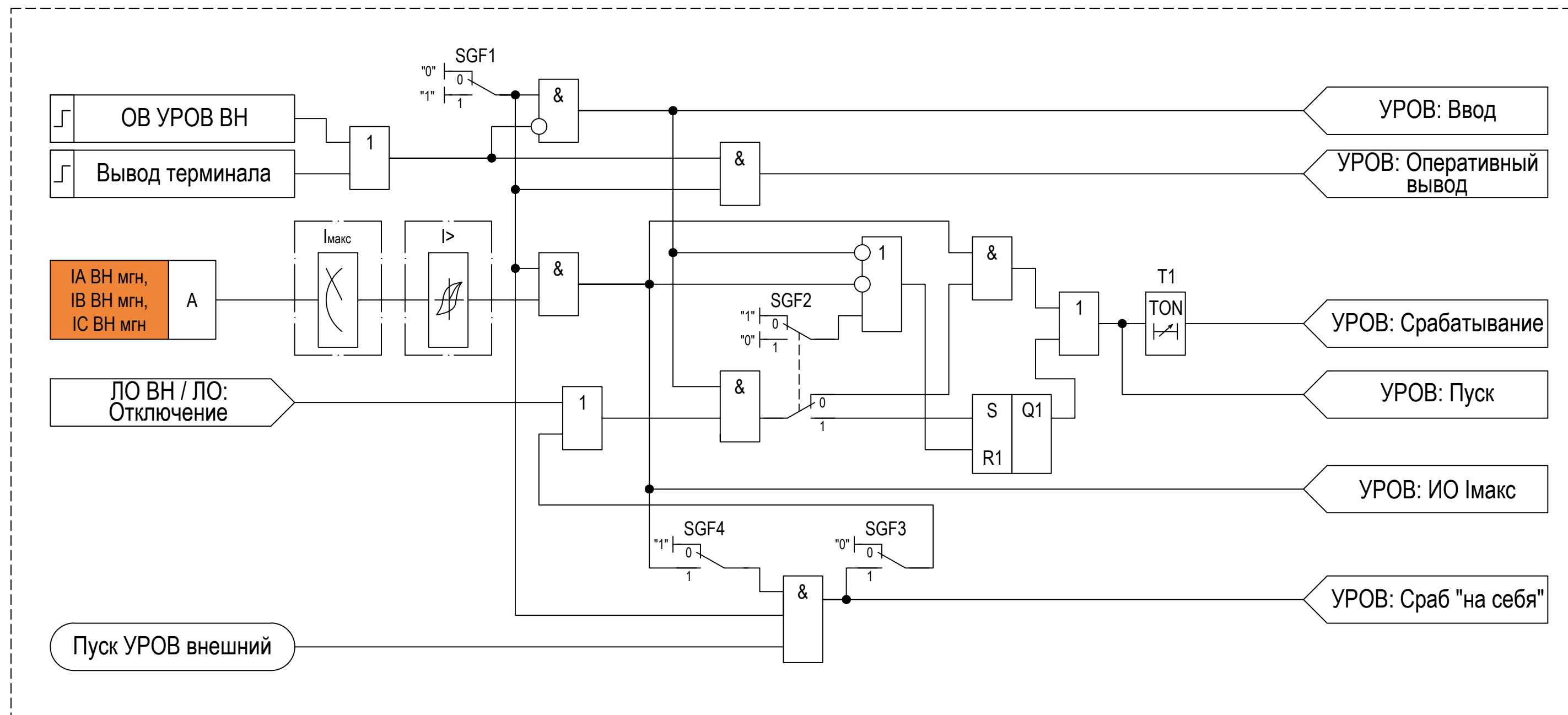
Устройство резервирования при отказе выключателя (УРОВ) (TPRBRF) RBRF1
